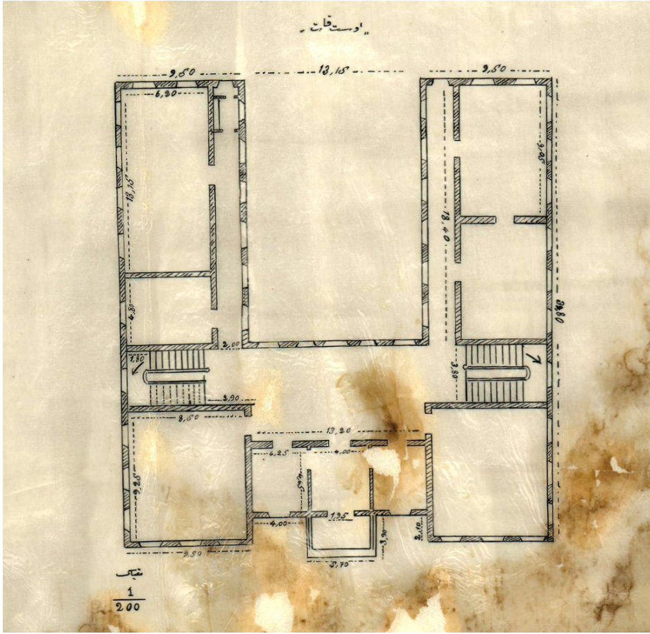
Şekil 4: Samsun Orta Mektebi Üst (Birinci) Kat Planı (T.C. Cumhurbaşkanlığı Devlet Arşivleri Başkanlığı Cumhuriyet Arşivi, 180.9.0.0. 98/477/2).
