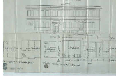
Çizim 24. Balıkesir kasabasında Karaoğlan Mahallesi'ndeki yanan Ermeni Mektebi'nin inşası için hazırlanmış olan plan. (Kaynak: BOA., İ.AZN., 49/22, 8 Zilkade 1320, 6 Şubat 1903).
